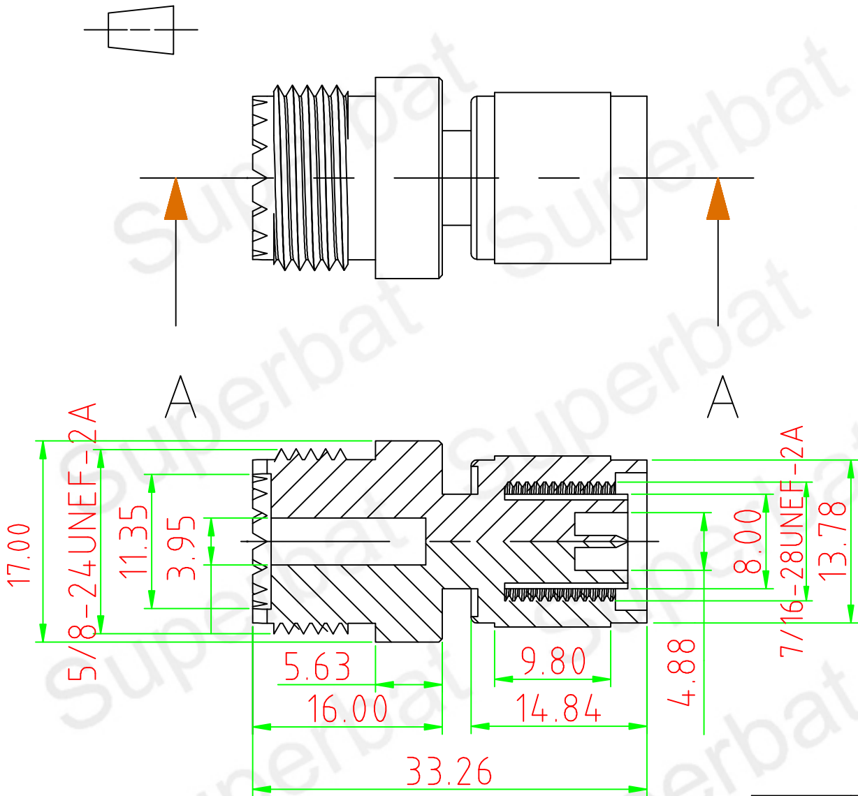
SECTION A-A
