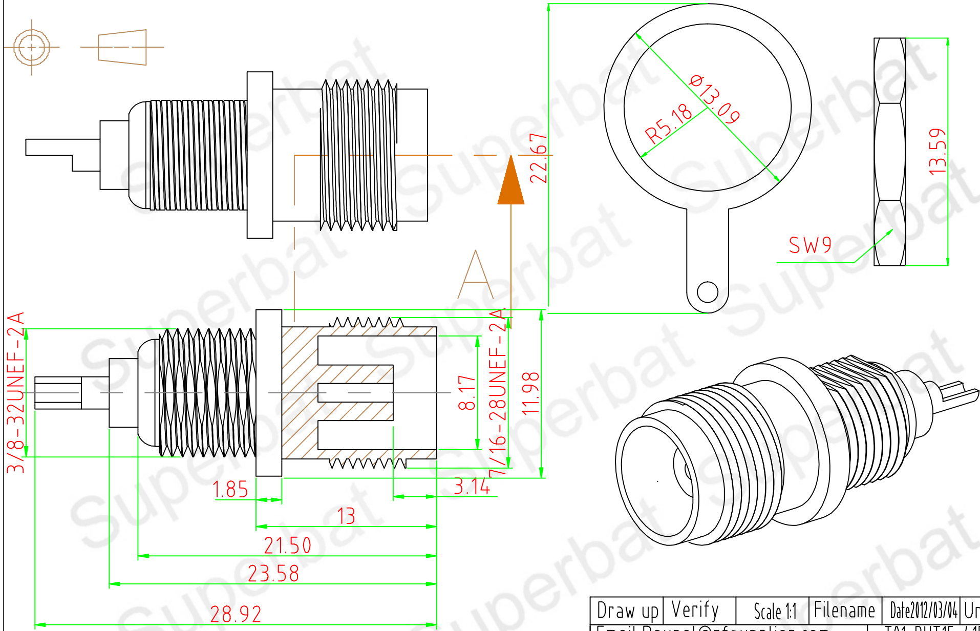
SECTION A-A
